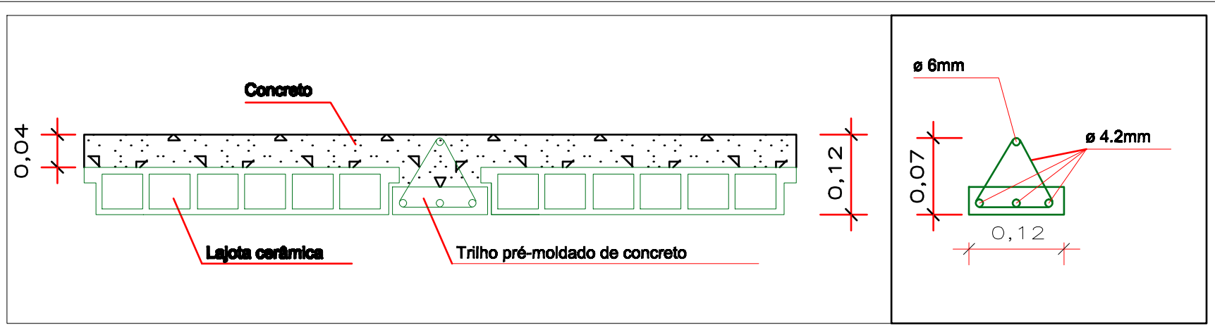
Detalhe da Laje Sem Escala
